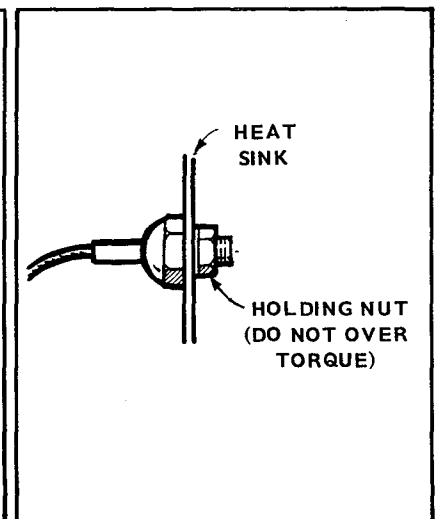
FIGURE 4-6. INSTALLING NEW RECTIFIERS
